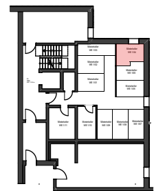
Kellergrundriss MSTB 1:500
